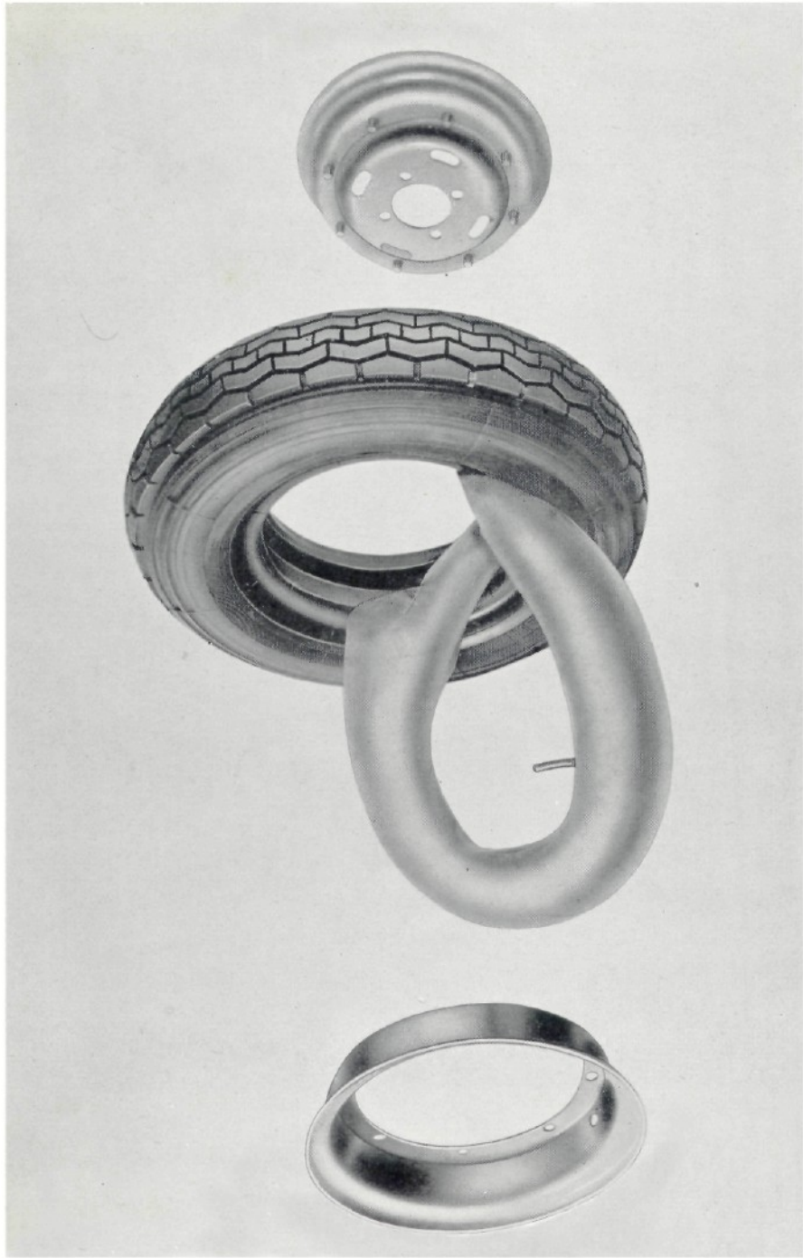
Fig. 17 - Smontaggio del pneumatico
