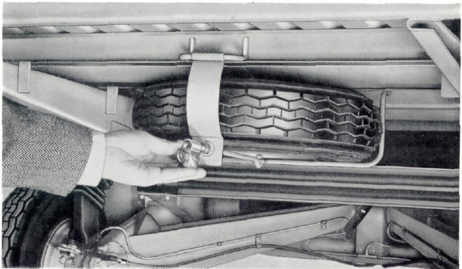
Fig. 16 - Fissaggio ruota scorta nel cestello
